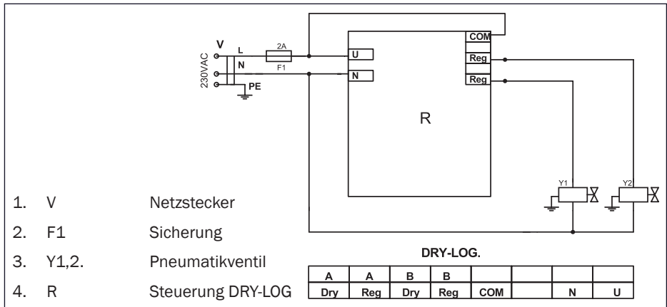
Abb.3.6.1. Elektroschaltplan
