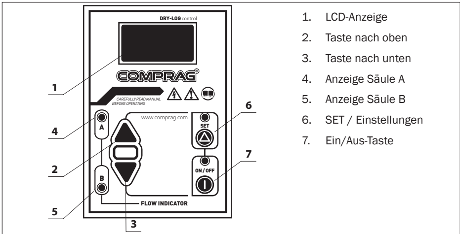
Abb. 4.1. Comprac DRY-LOG Steuerung
