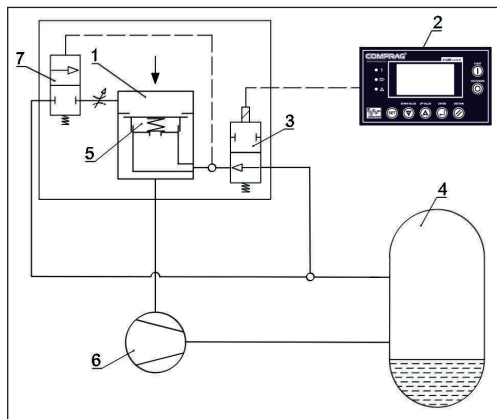
Рис. 2.5 Система регулировки
