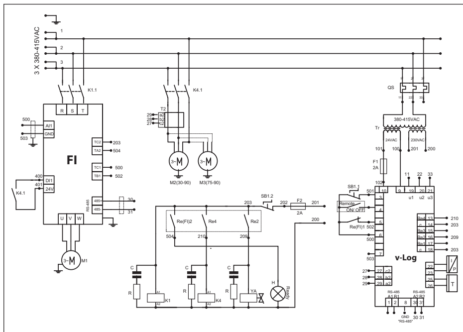
Рис. 2.6.1 Схема электрическая DV11 – DV22
