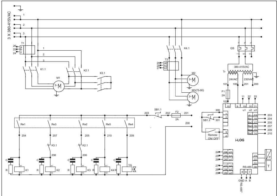
Bild 2.6 Elektro-Schaltplan A75-90
