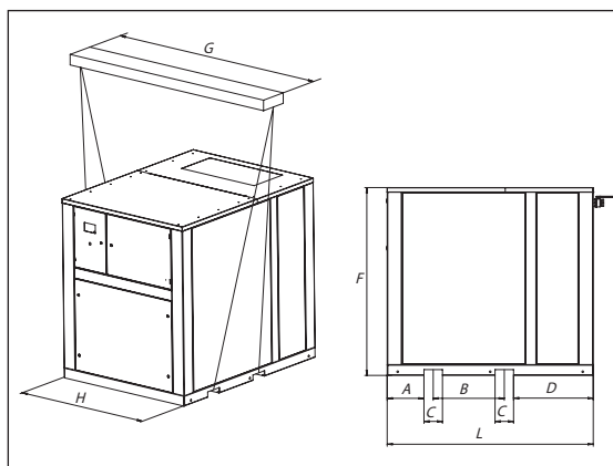
Рис. 3.1 Схема для такелажных работ A75-90
